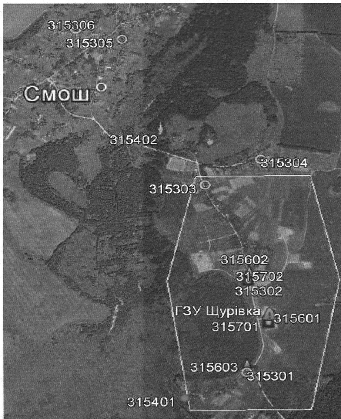
Рисунок 1 - Розташування пунктів відбору проб ОНПС в межах Щурівського нафтового родовища
